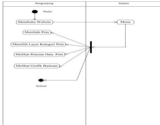
Gambar 3. Activity Diagram Pengunjung
