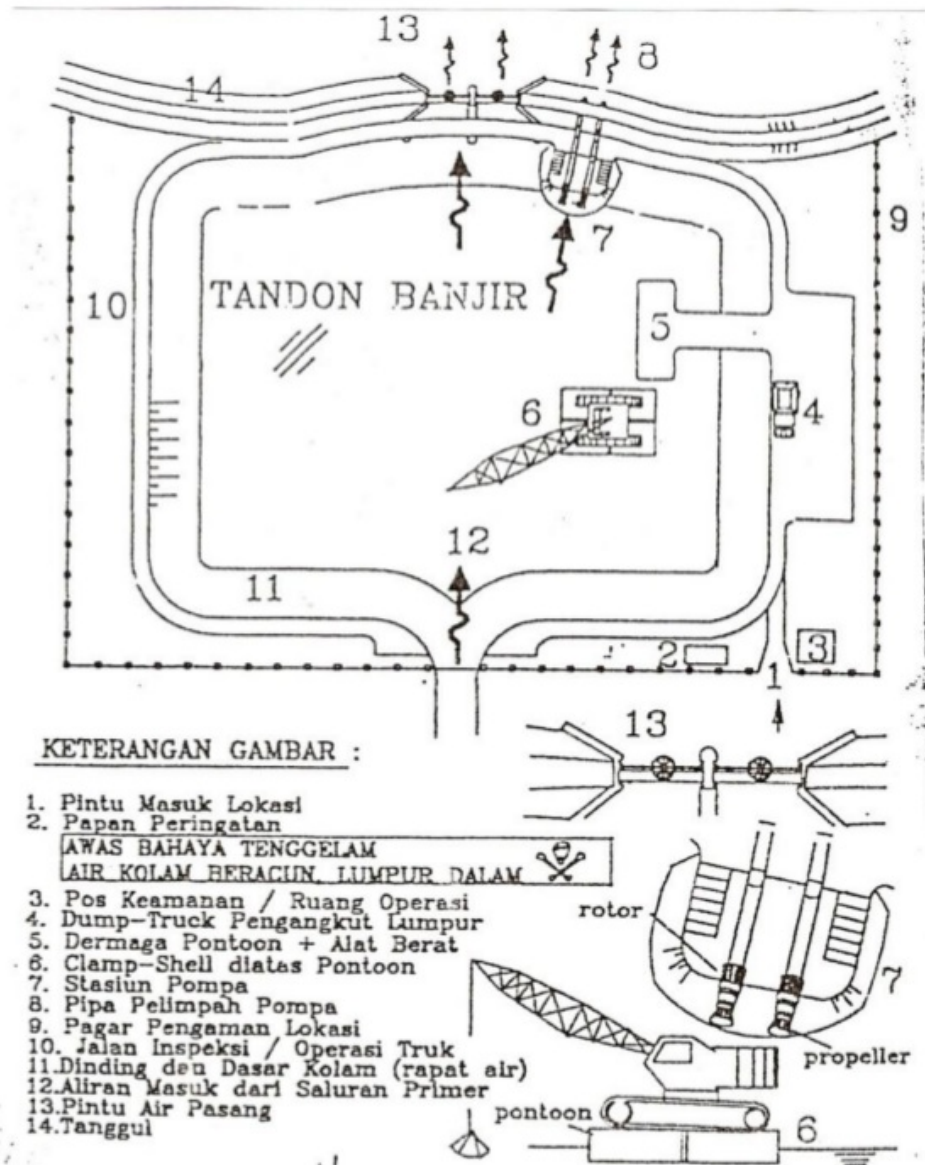
Gambar 7.5. Tandon Banjir
