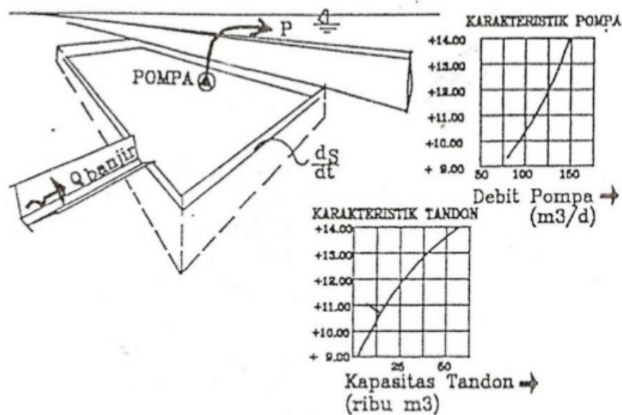
Gambar 7.4. Tandon banjir dengan Pompa Sentrifugal
