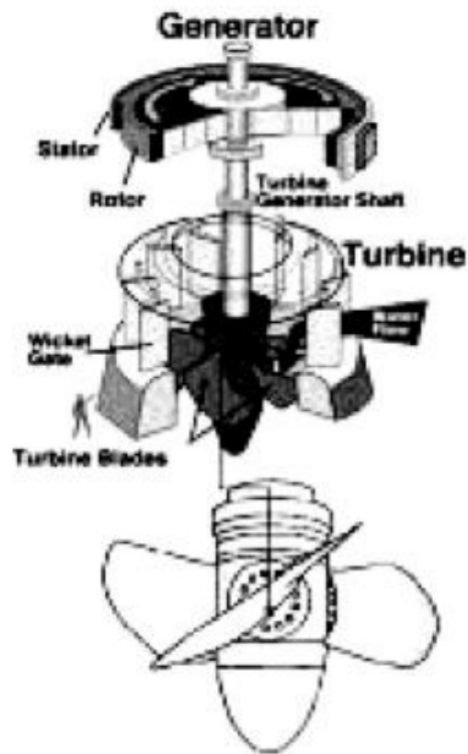
Gambar 2. Jenis turbin kaplan
