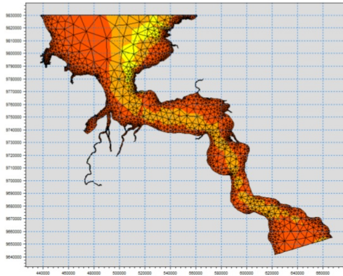
Gambar 2. Model jaring kisi-kisi di selat Bangka
