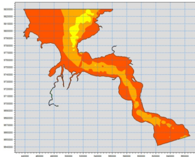
Gambar 3. Batimetri model global untuk daerah selat Bangka
