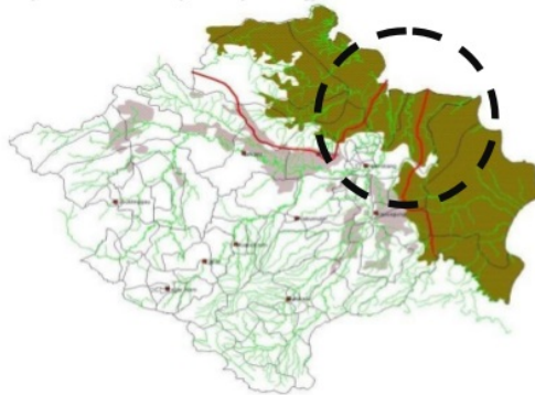
Gambar 1. Peta Lokasi Penelitian (Sumber: BPSDA, 2010)
