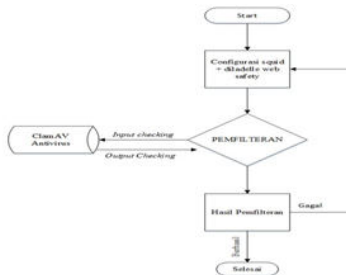
Gambar 4: Flowchart Pengujian
