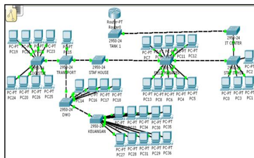
Gambar 3.1 Topologi PT. Pertamina UbeP Adera Pengabuan
