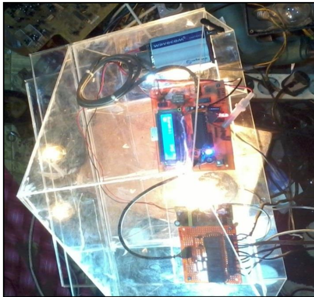
Gambar 8. Sistem pengedali lampu dalam keadaan aktif
