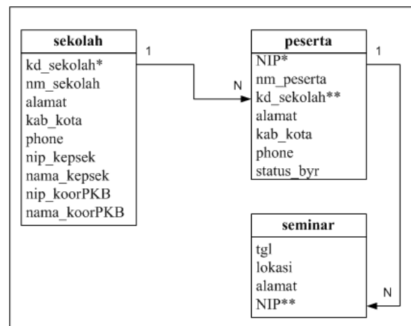
Gambar 4. Relasi antar Tabel
