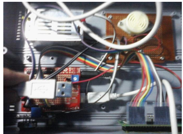
Gambar 5.5 Kabel USB dihubungkan dengan Arduino Uno
