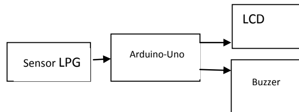
Gambar 4.13. Skema Rangkaian Lengkap Alat Pendeteksi Kebocoran Gas LPG
