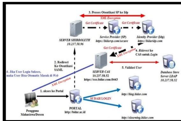
Gambar 2. Arsitektur Sistem
