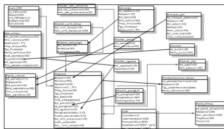
Gambar 2: Metodologi Penelitian
