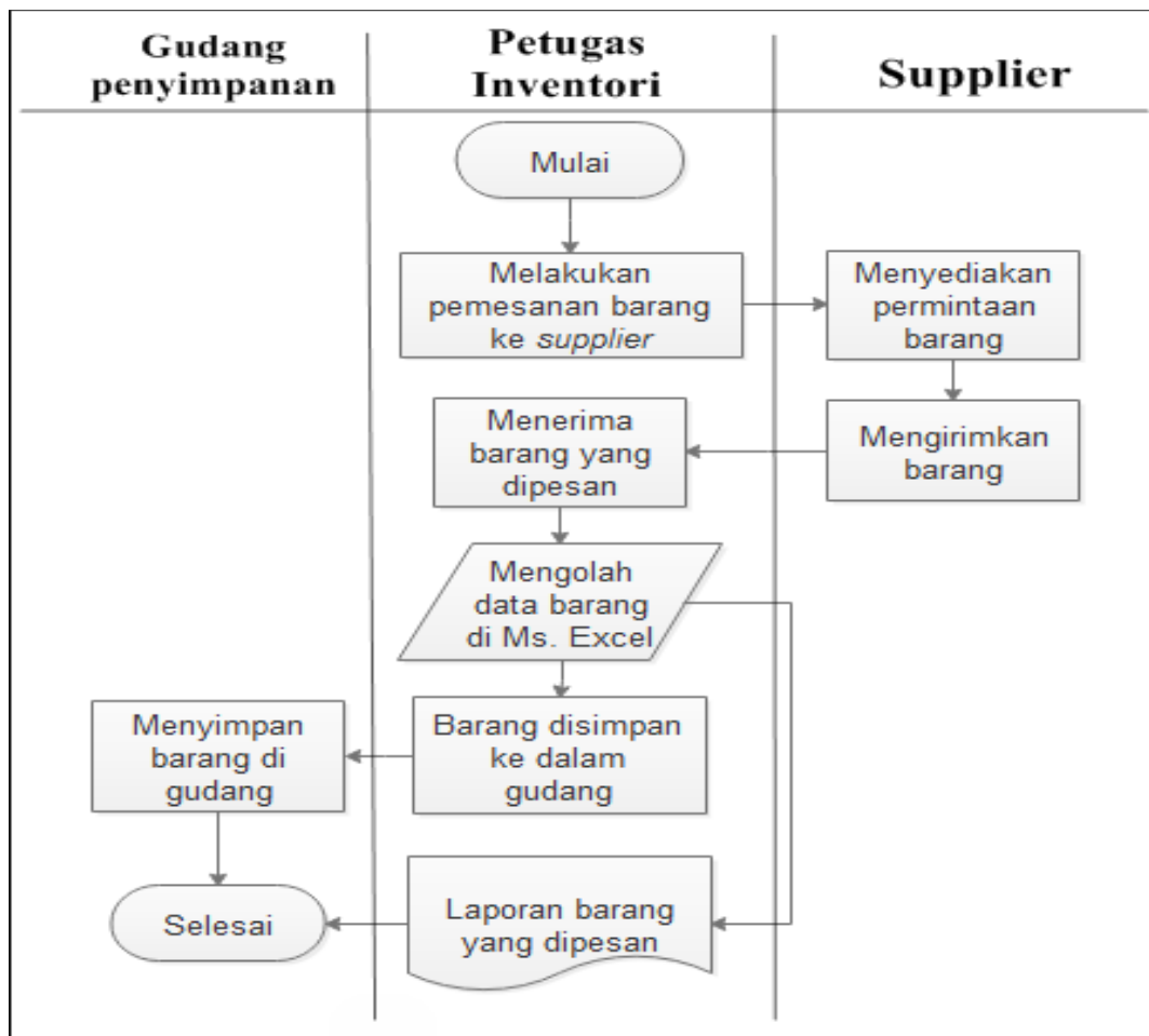
Gambar 4.1 Flowchart Sistem yang Sedang Berjalan (Barang Masuk)
