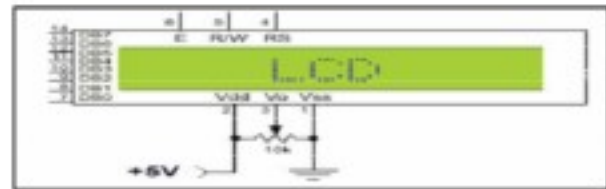
Gambar 4 Rangkaian LCD
