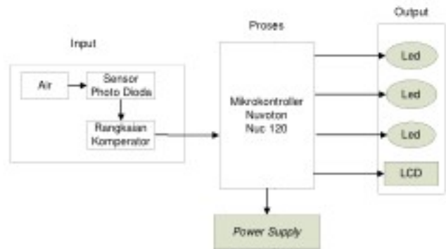
Gambar 7 Blok Diagram Rangkaian
