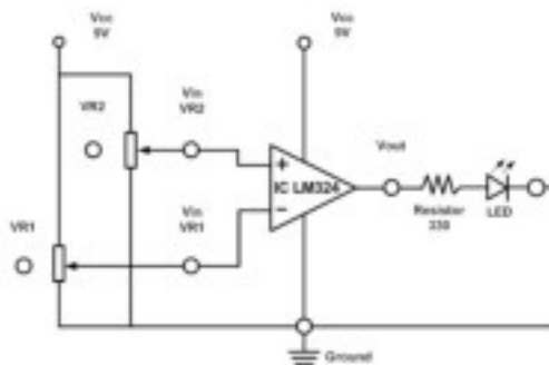
Gambar 2 Rangkaian komparator
