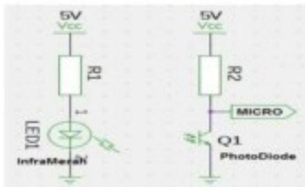
Gambar 1. Gambar Rangkaian Sensor.
