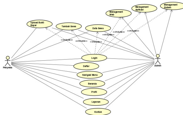
Gambar. 2 Usecase Putri Tenda
