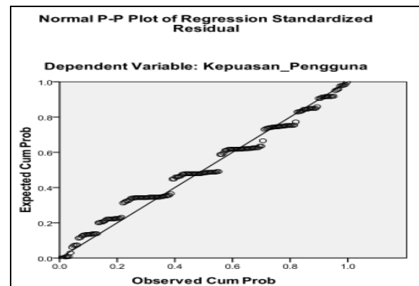
Gambar 1. Uji Normalitas
