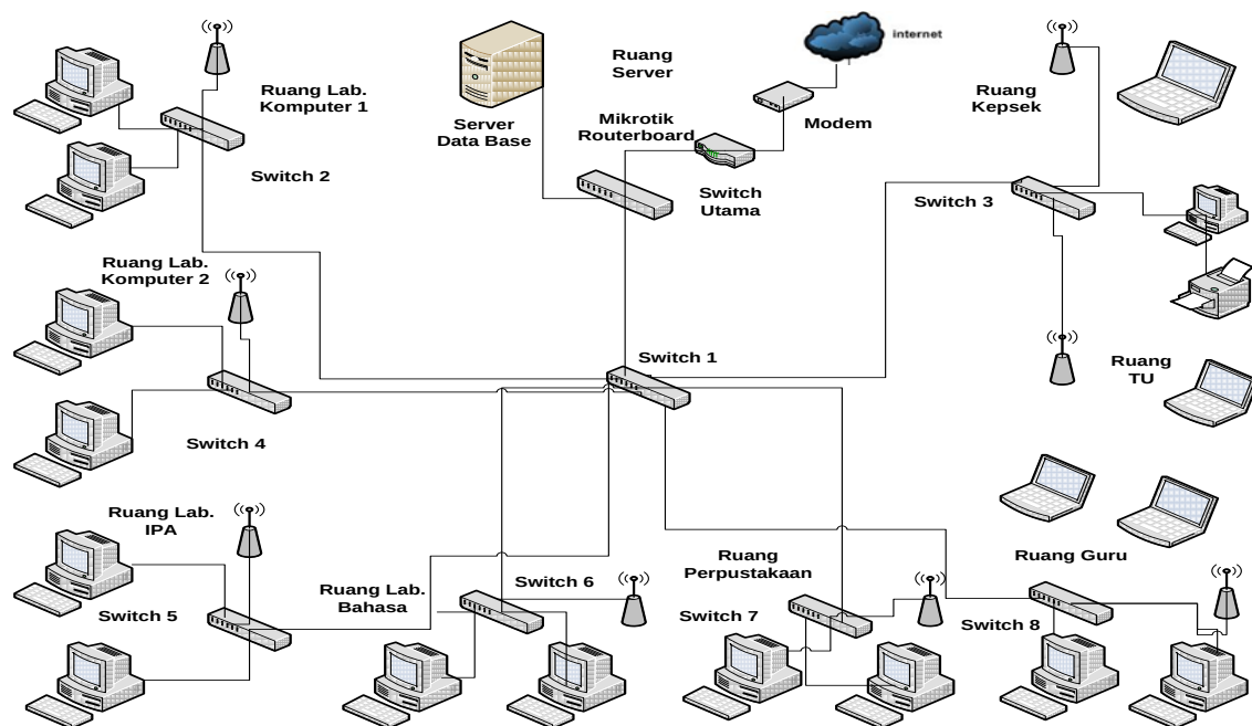
Gambar 5. Perancangan Topologi Jaringan SMA Negeri 1 Indralaya Selatan
