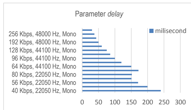
Gambar 4. Grafik hasil pengamatan parameter delay
