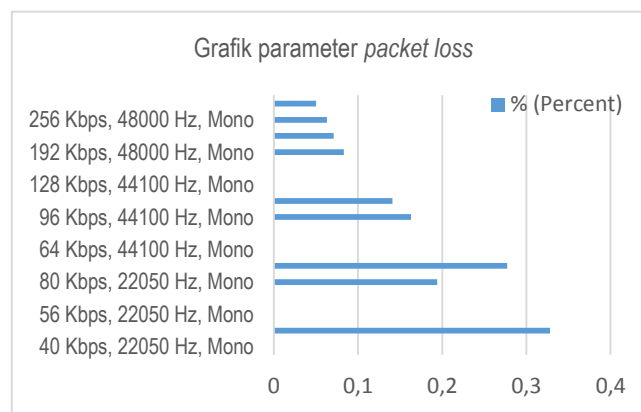
Gambar 5. Grafik pengujian parameter packet loss
