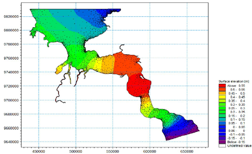
Gambar 2. Model hidrodinamika elevasi permukaan aliran sungai
