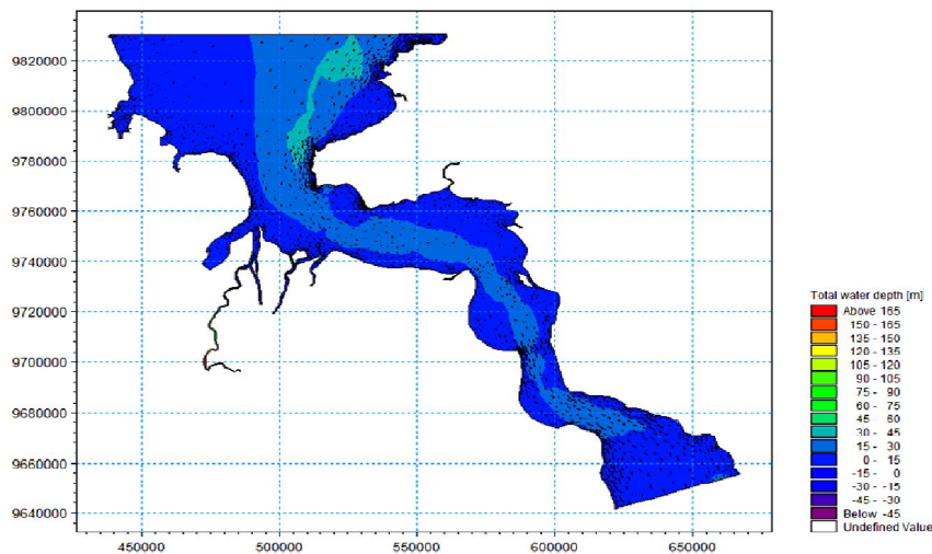
Gambar 3. Model hidrodinamika total kedalaman aliran sungai
