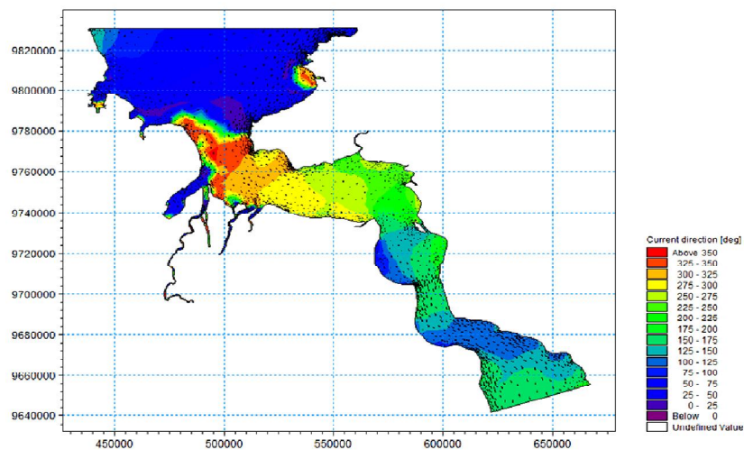
Gambar 1. Model hidrodinamika arah kecepatan air sungai
