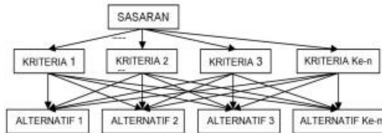
Gambar 1 Struktur AHP (4)
