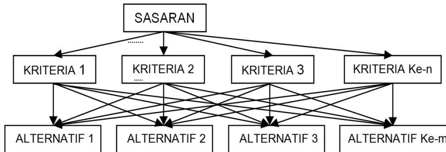
Gambar 1 Struktur AHP (4)
