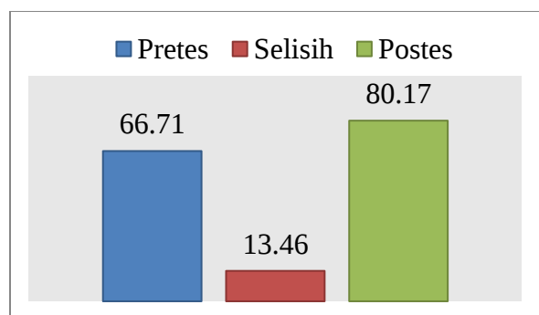
Diagram 2 Rata-Rata Nilai Pretes dan Postes Menulis
