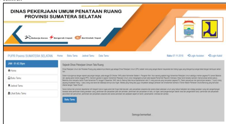
Gambar 4. Tampilan utama
