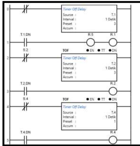
Gambar 8. Ladder diagram Belt Conveyor pada Outseal PLC
