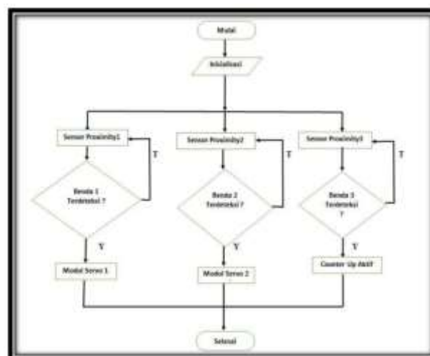
Gambar 5. Flow Chart pemilah otomatis pada belt conveyor
