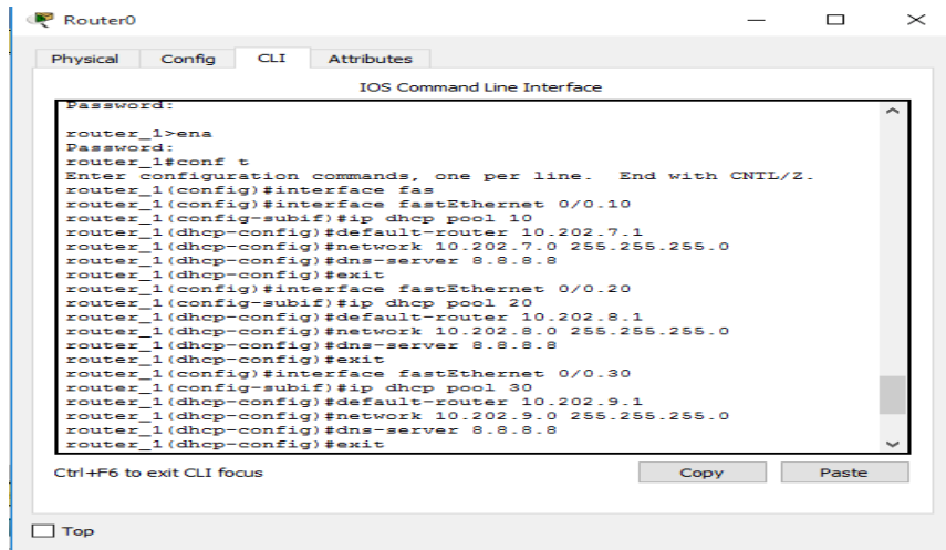
Gambar 4. Konfigurasi DHCP
