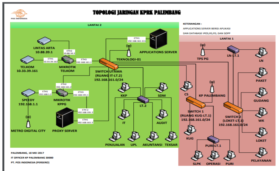
Sumber : Kepala IT PT. Pos Indonesia Palembang. Gambar 2. Topologi jaringan PT Pos Indonesia Palembang.
