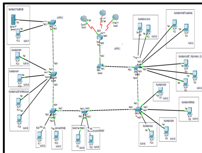
Gambar 4. Rancangan topologi manajemen vlan
