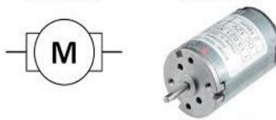
Gambar 7. Simbol dan Bentuk Fisik Motor DC
