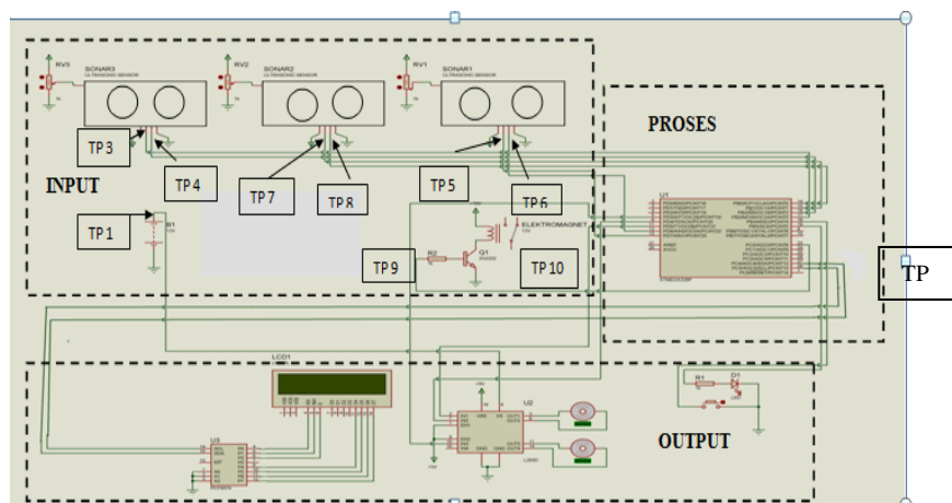
Gambar 12. Titik Pengukuran Pada Skema Rangkaian
