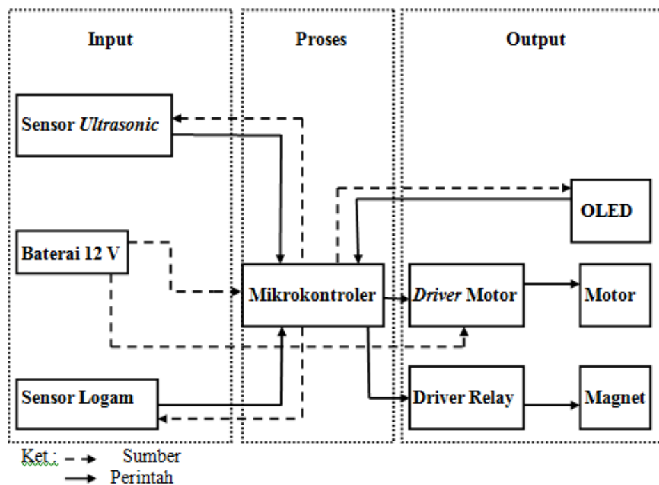
Gambar 1. Blok Diagram Robot Pendeteksi Logam Dengan Mikrokontroler
