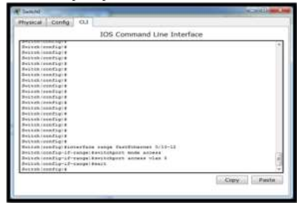
Gambar 14. Konfigurasi switchport VLAN 5
