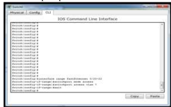
Gambar 16. Konfigurasi switchport VLAN 7
