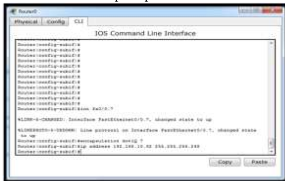
Gambar 25. Konfigurasi interface VLAN 7 pada Router
