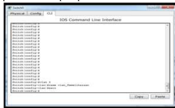
Gambar 4. Konfigurasi vlan pemeliharaan
