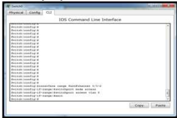
Gambar 17. Konfigurasi switchport VLAN 8
