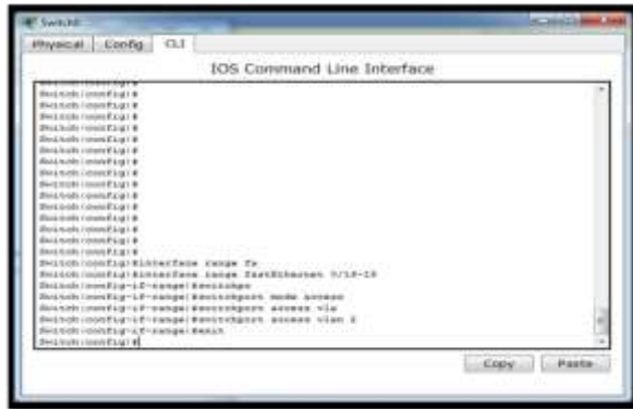
Gambar 11. Konfigurasi switchport VLAN 2
