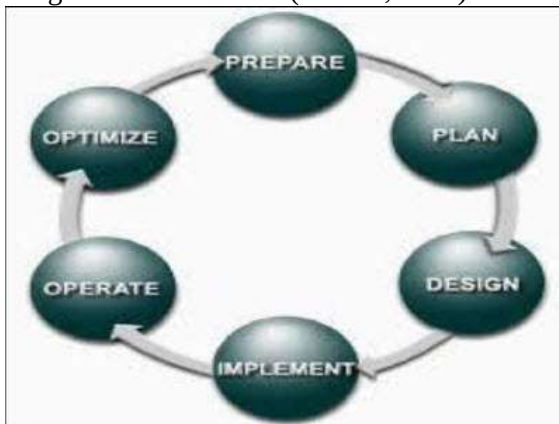
Gambar 1. Metode PPDIOO
