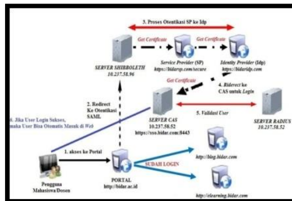
Gambar 2. SSO dengan SAML Berbasis Radius
