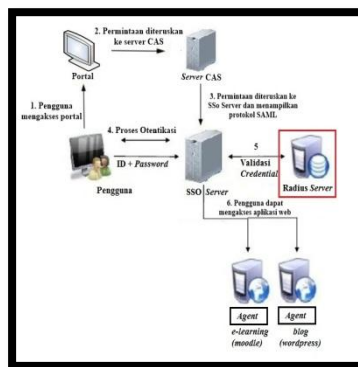
Gambar 1. Model Arsitektur Sistem
