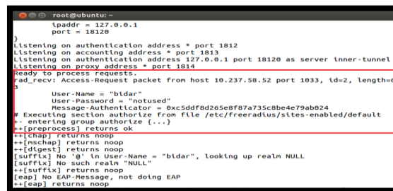
Gambar 4. LogFreeradius Berhasil
