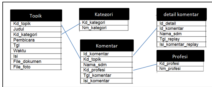
Gambar 3. Rancangan Database
