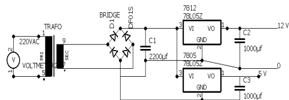
Gambar 7 Rangkaian Catu Daya
