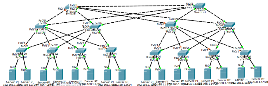
Gambar 2: TSimulasi canonical tree DC.
