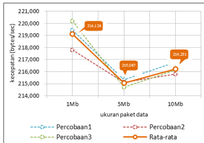
Gambar 7: Hasil uji kecepatan transfer data pada topologi Folded Clos Tree (kondisi normal).
