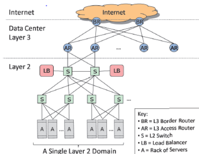
Gambar 1: Arsitektur jaringan konvensional untuk pusat data (diadaptasi dari gambar oleh Cisco (Cisco systems. 2004)
