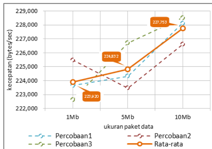
Gambar 6: Hasil uji kecepatan transfer data pada topologi Canonical Tree (kondisi normal).
