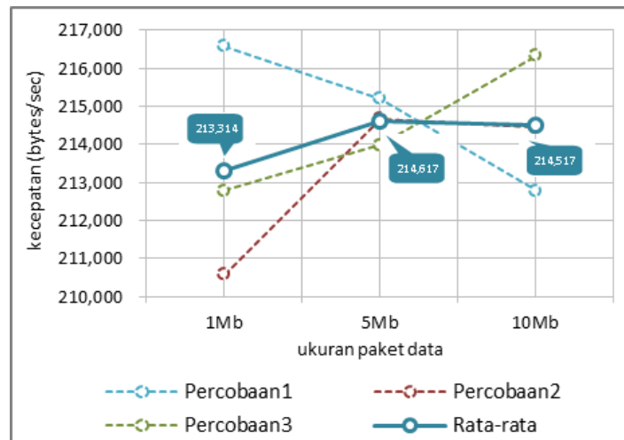
Gambar 9: Hasil uji kecepatan transfer data pada topologi Folded Clos Tree (kondisi terdapat gangguan).
