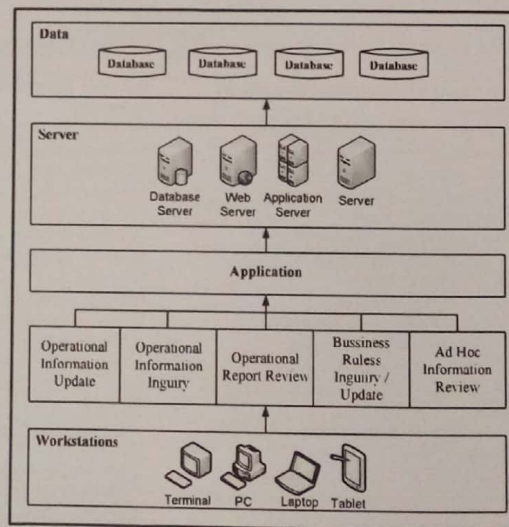
Gambar 4. Arsitektur Sistem Bisnis Konseptual
