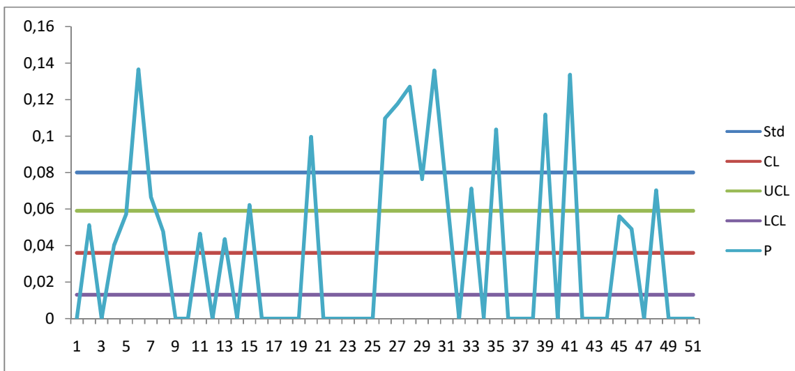
Gambar 1. Peta kendali P bulan Januari – Februari 2018
