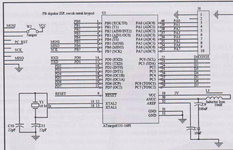
Gambar 2. Rangkaian Mikrokontroler ATMega16
