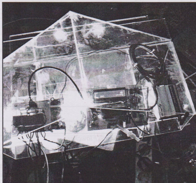
Gambar 7. Tampilan Atas Sistem Pengendali Lampu
