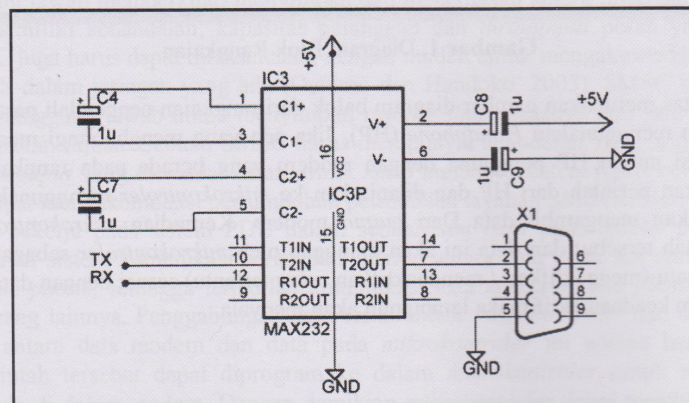
Gambar 3. Koneksi Port dengan Modem
