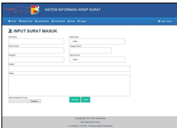
Gambar 11. Formulir Input Surat Masuk
