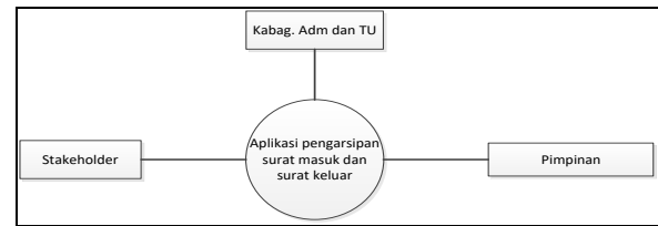
Gambar 2. Diagram Konteks
