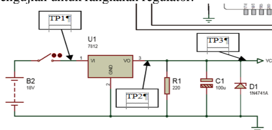
Gambar 6. Titik Pengujian Rangkaian Regulator
